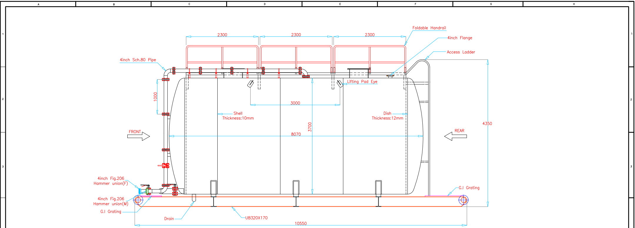
ELEVATION
